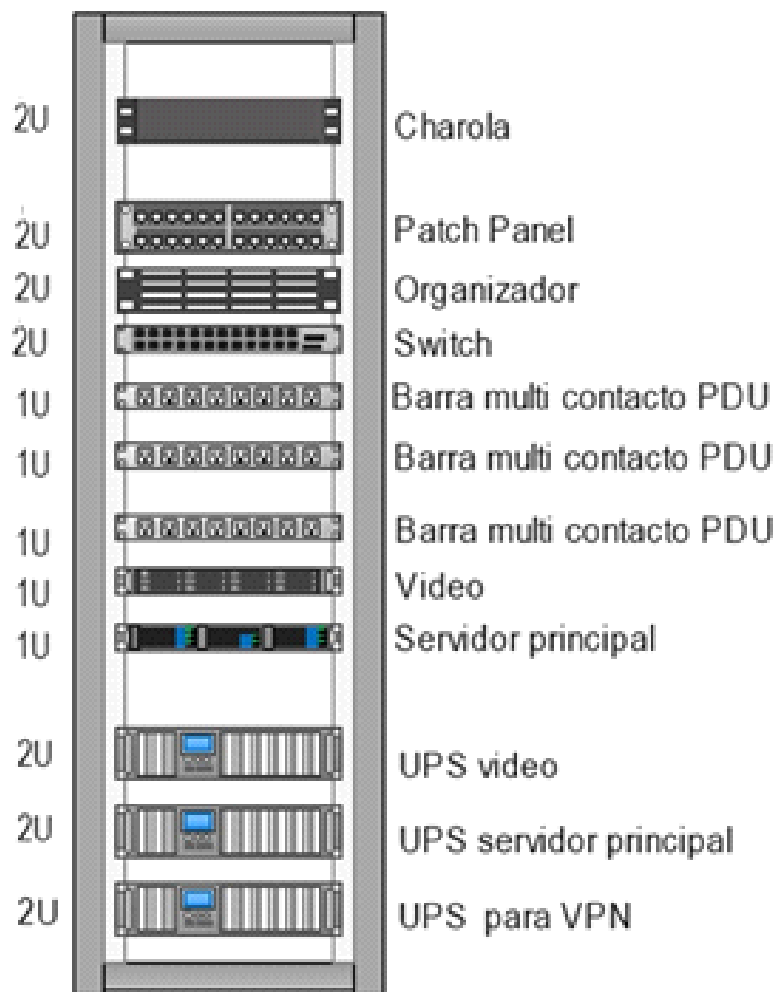
Figura 4.11 Ejemplo de la disposición del gabinete central.
