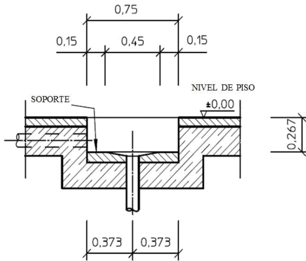
Figura 4.2 Diagrama de instalación del dinamómetro, vista lateral.
