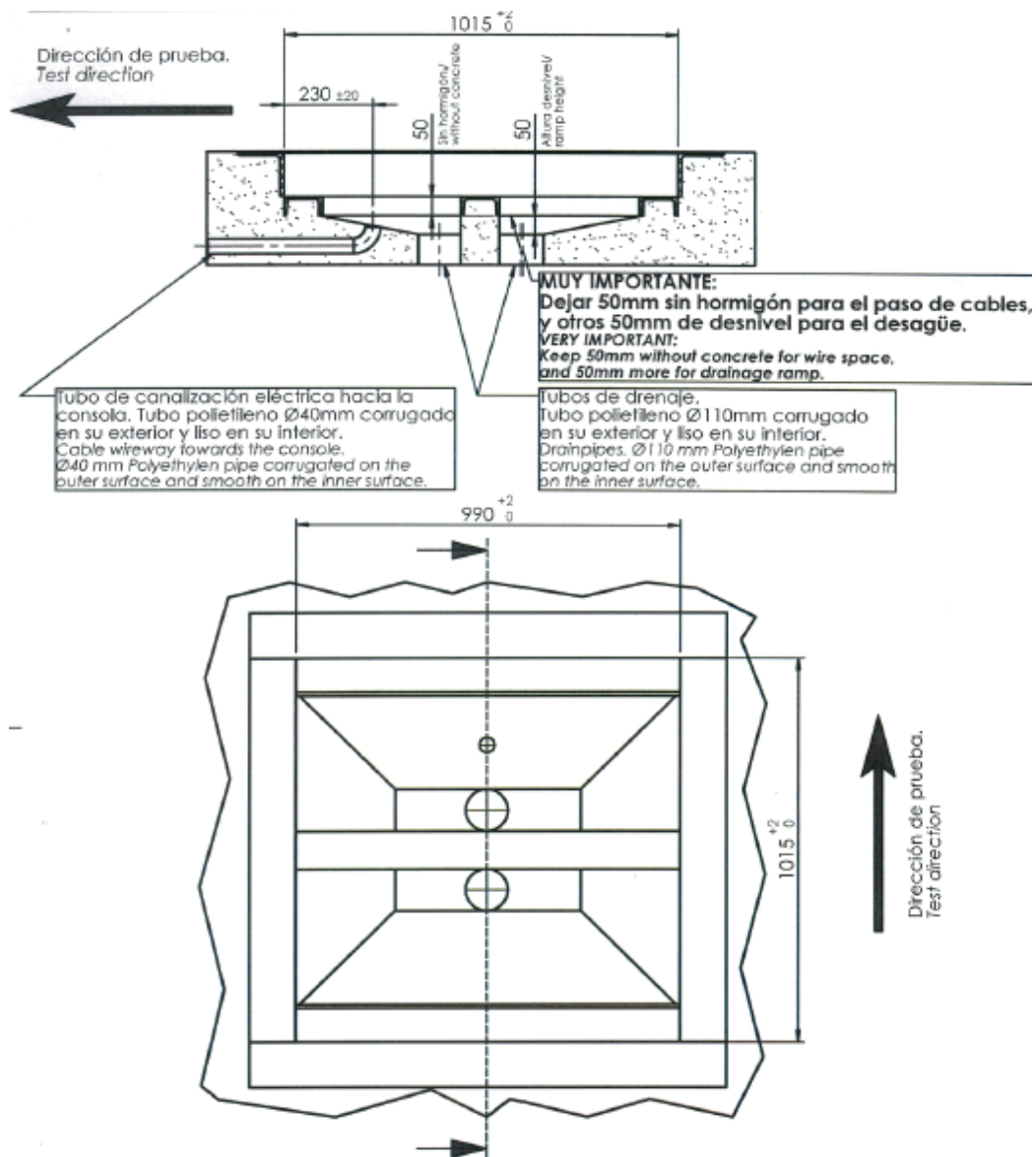
Figura 4.8 Fosa para la instalación de los equipos de inspección físico-mecánica, alineador al paso.
