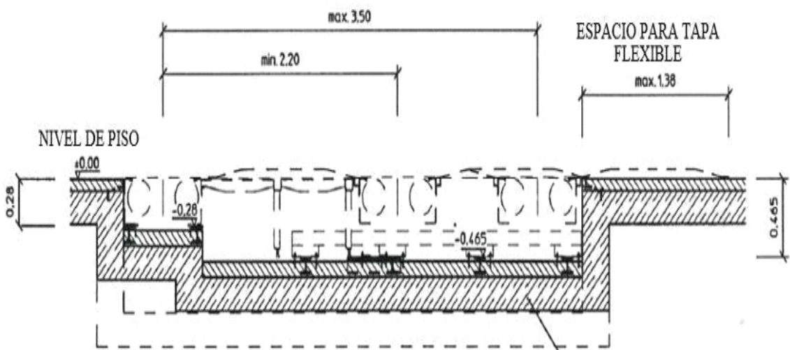
Figura 4.5 Diagrama de instalación del dinamómetro para vehículos de doble tracción, vista lateral (sección A-A).
