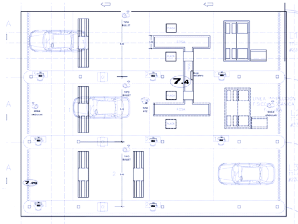
Figura 7.2 Ejemplo de disposición de las cámaras de video vigilancia en las líneas de Verificación Vehicular.
