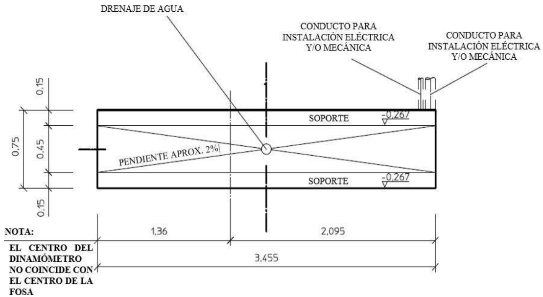
Figura 4.3 Diagrama de instalación del dinamómetro, vista superior.
