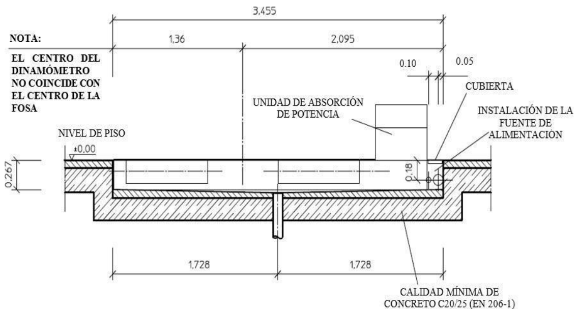
Figura 4.1 Diagrama de instalación del dinamómetro, vista frontal.
