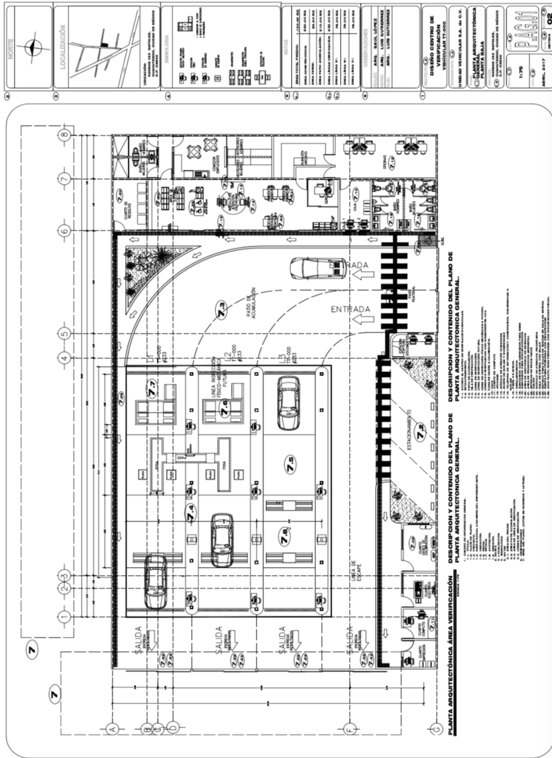
Figura 3.7. Ejemplo de plano del Centro de Verificación Vehicular. Nótese que esta imagen se presenta como ejemplo, y puede no incluir todos los elementos mínimos que requieran las autoridades competentes.
