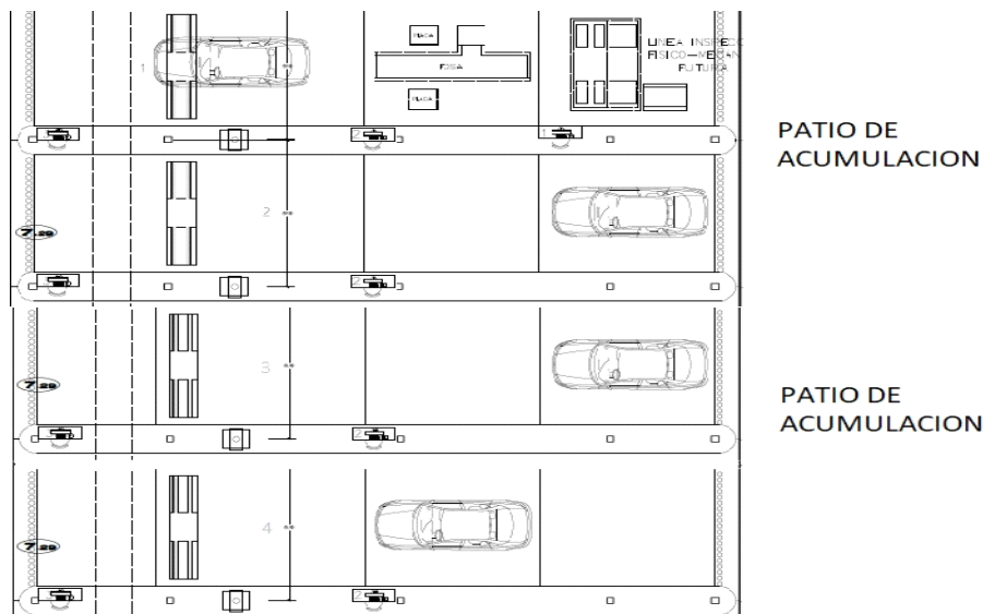
Figura 3.2. Modelo de Centro con un área de verificación.
