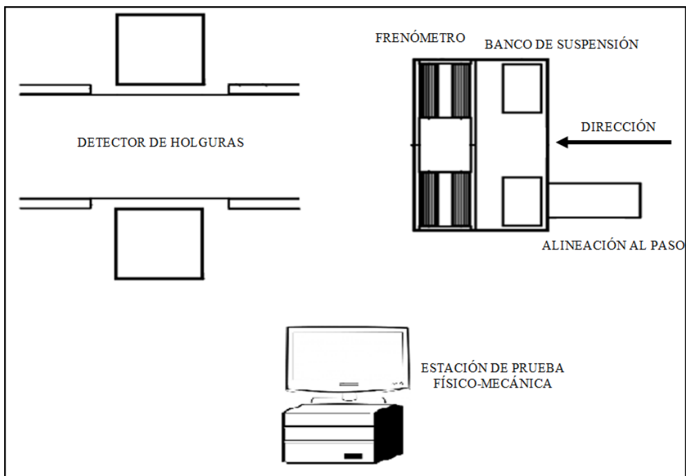
Figura 4.18 Ubicación de la estación de prueba físico-mecánica.
