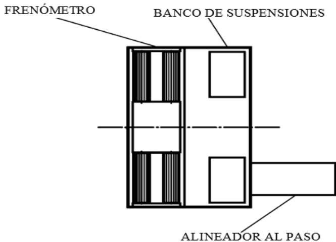
Figura 4.13 Instalación de los equipos alineador al paso, banco de suspensiones y frenómetro.
