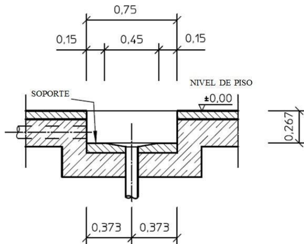
Figura 4.5 Diagrama de instalación del dinamómetro, vista lateral.
