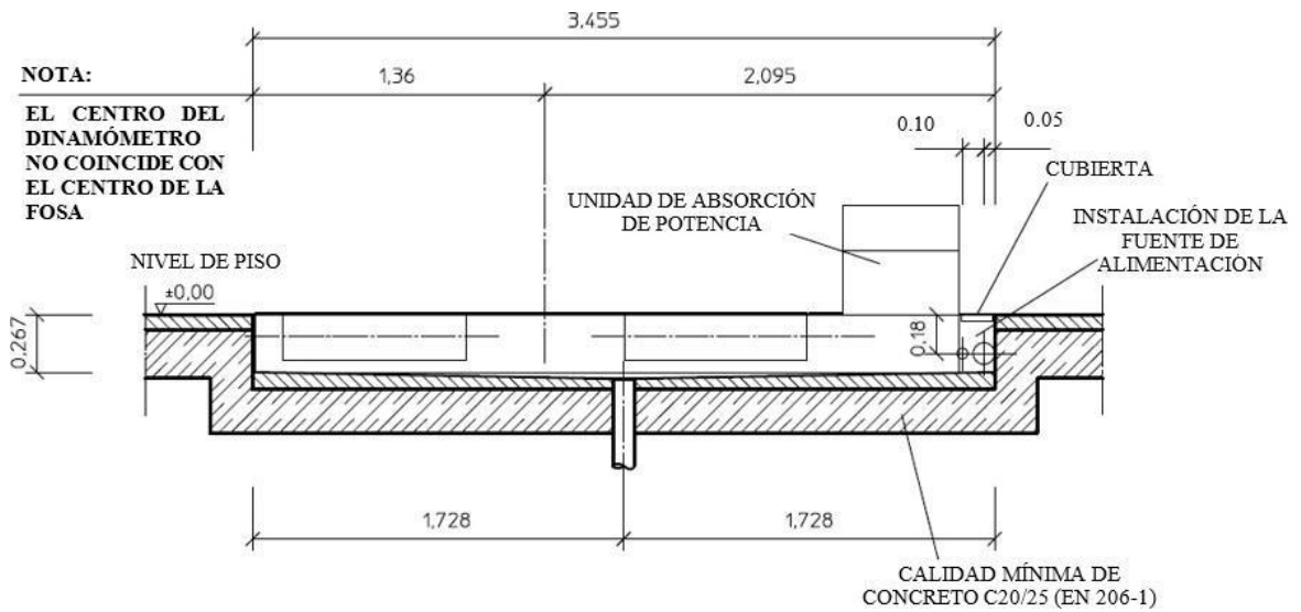
Figura 4.4 Diagrama de instalación del dinamómetro, vista frontal.
