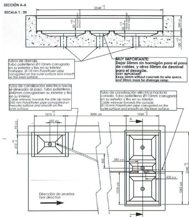
Figura 4.14 Fosa para la instalación de los equipos de inspección físico-mecánica, alineador al paso.
