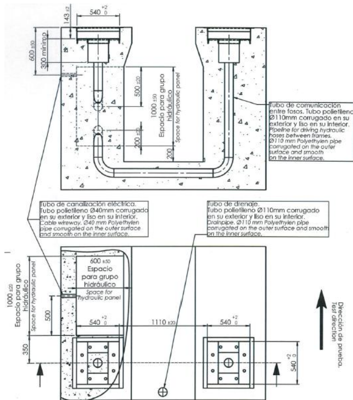
Figura 4.16 Diagrama de la fosa de inspección de Detector de Holguras.
