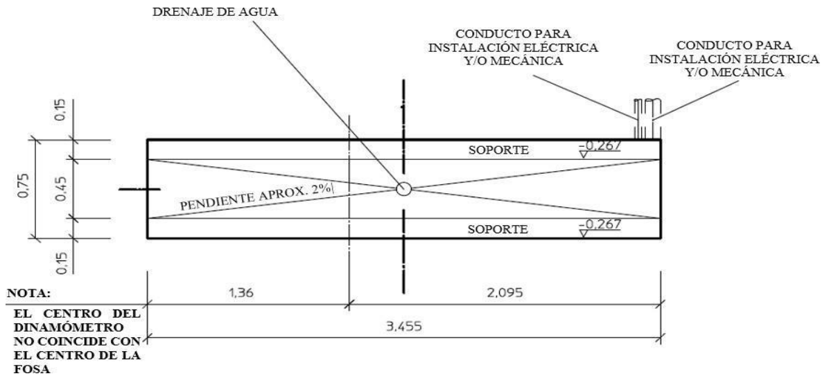
Figura 4.6 Diagrama de instalación del dinamómetro, vista superior.
