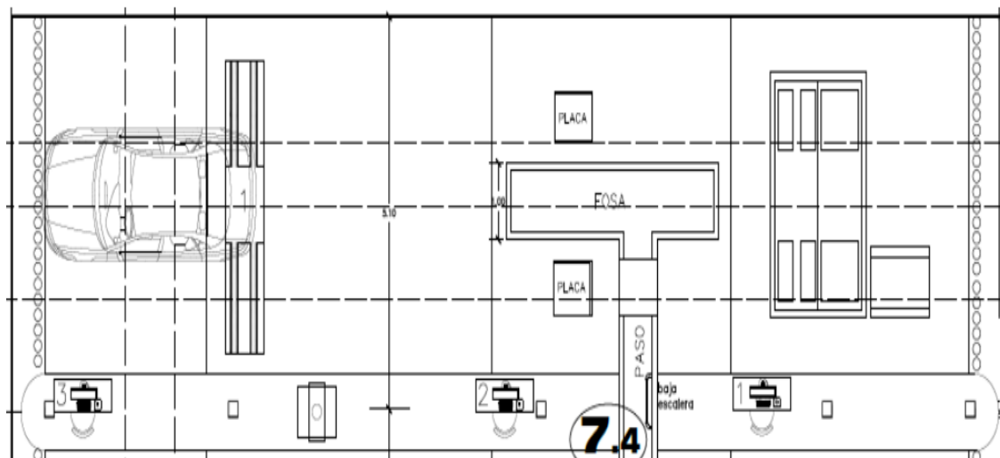
Figura 3.3 Línea de Verificación Vehicular.
