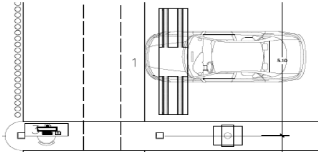
Figura 3.5 Línea de medición de emisiones contaminantes con dinamómetro para vehículos de tracción delantera.
